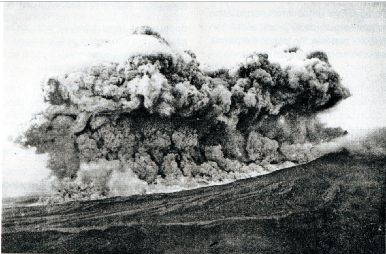
nuée ardente
