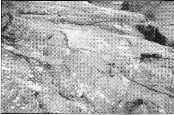
Photo 18 - Plate-forme prismée du premier niveau.
