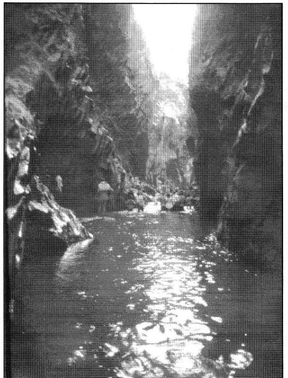
Photo 22 - Gorges d'Alcantara, Sicile.
