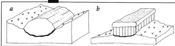
Schéma 3 - a. Mise en place dans une vallée fluviale ; b. Inversion de relief après phase d'érosion.
