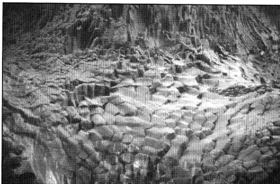
Photo 24 - Gorges d'Alcantara, Sicile, érosion des prismes.
