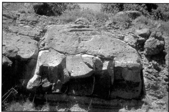
Photo 14 - Coulée de Baldy-Batipaume, Le Cap-d'Agde.
