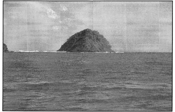
Photo 20 - Ilots du Robert.
