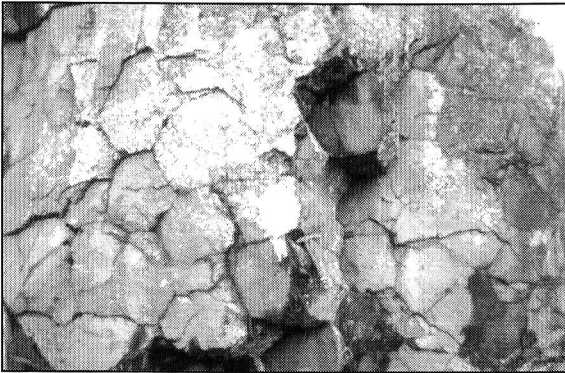
Photo 19 - Paroi verticale, bord du centre du culot.
