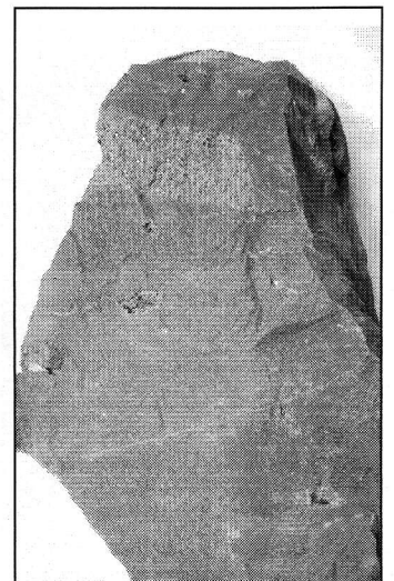
Photos 12 et 13 - Saint-Jean-le-Centenier, Coirons. Coulée prismée et échantillon avec enclave de péridotite.
