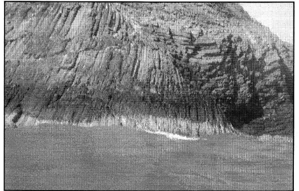
Photo 21 - Ilots du Robert, détail.
