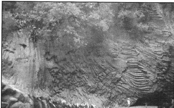
Photo 23 - Gorges d'Alcantara, Sicile.
