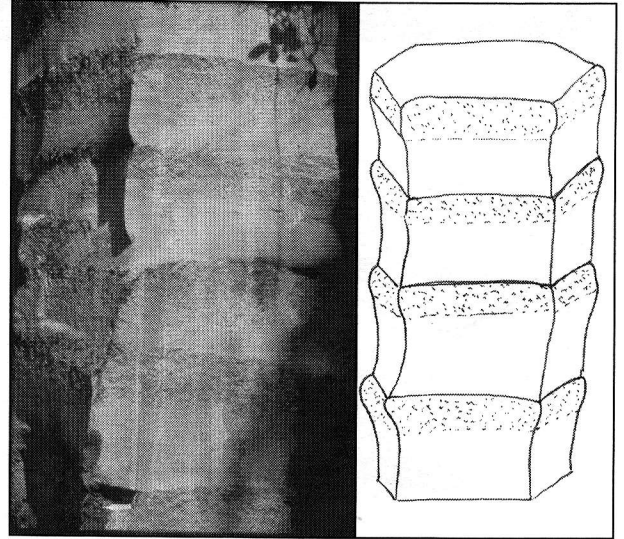
Photo 2 - Royat, grotte des Laveuses, près de Clermont-Ferrand.
