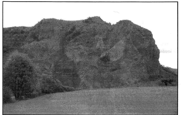
Photo 11 - Rocher de Laval, Neussargues, Cantal.
