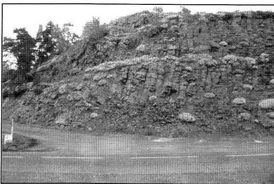
Photo 16 - Bournacle, Velay. Coulée prismée avec altération en boule des prismes.
